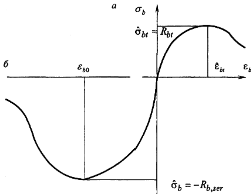
Рисунок 7 - Криволинейные диаграммы деформирования бетона
