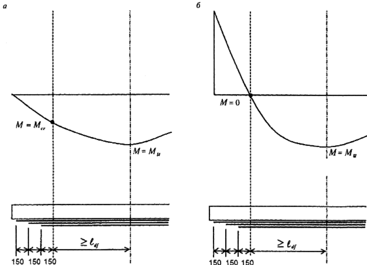
а - свободно опертый элемент; б - неразрезной элемент
