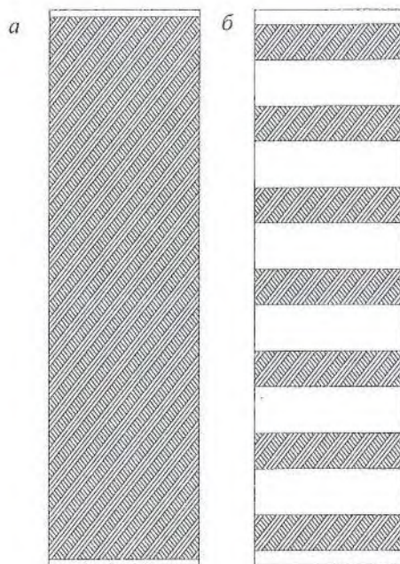
Рисунок 18 – Способы усиления колонн обоями
