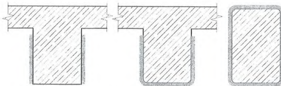
Рисунок 8 – Схемы усиления наклонных сечений элементов
