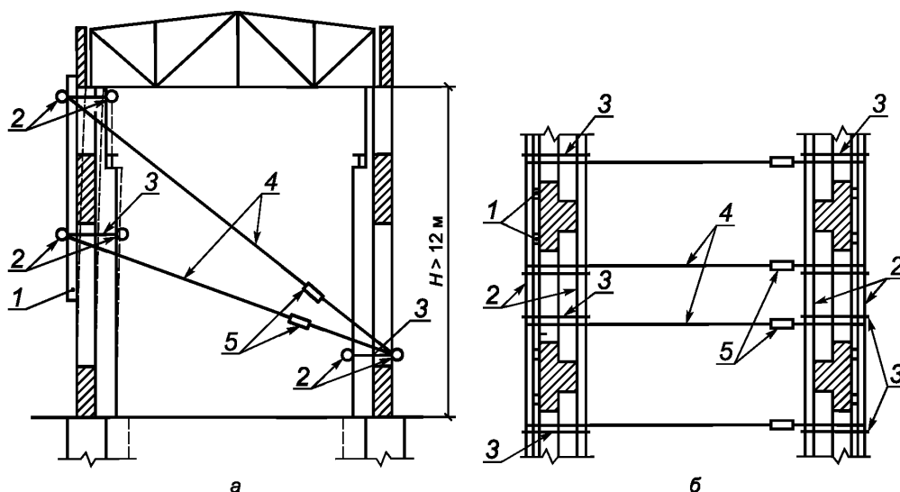
а — поперечное сечение; б — горизонтальное сечение; 1 — стойка; 2 — поперечина; 3 — проволоочные скрутки диаметром 5—6 см или стальные уголки; 4 — тяж диаметром 16 мм; 5 — натяжные муфты
