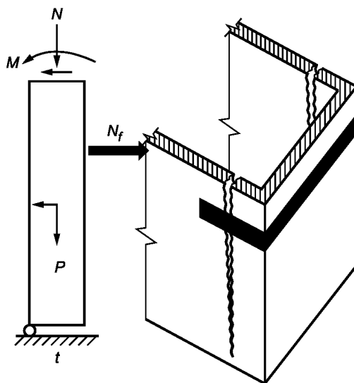
Рисунок 27 — Схема усиления кладки стены с трещинами от опрокидывания
