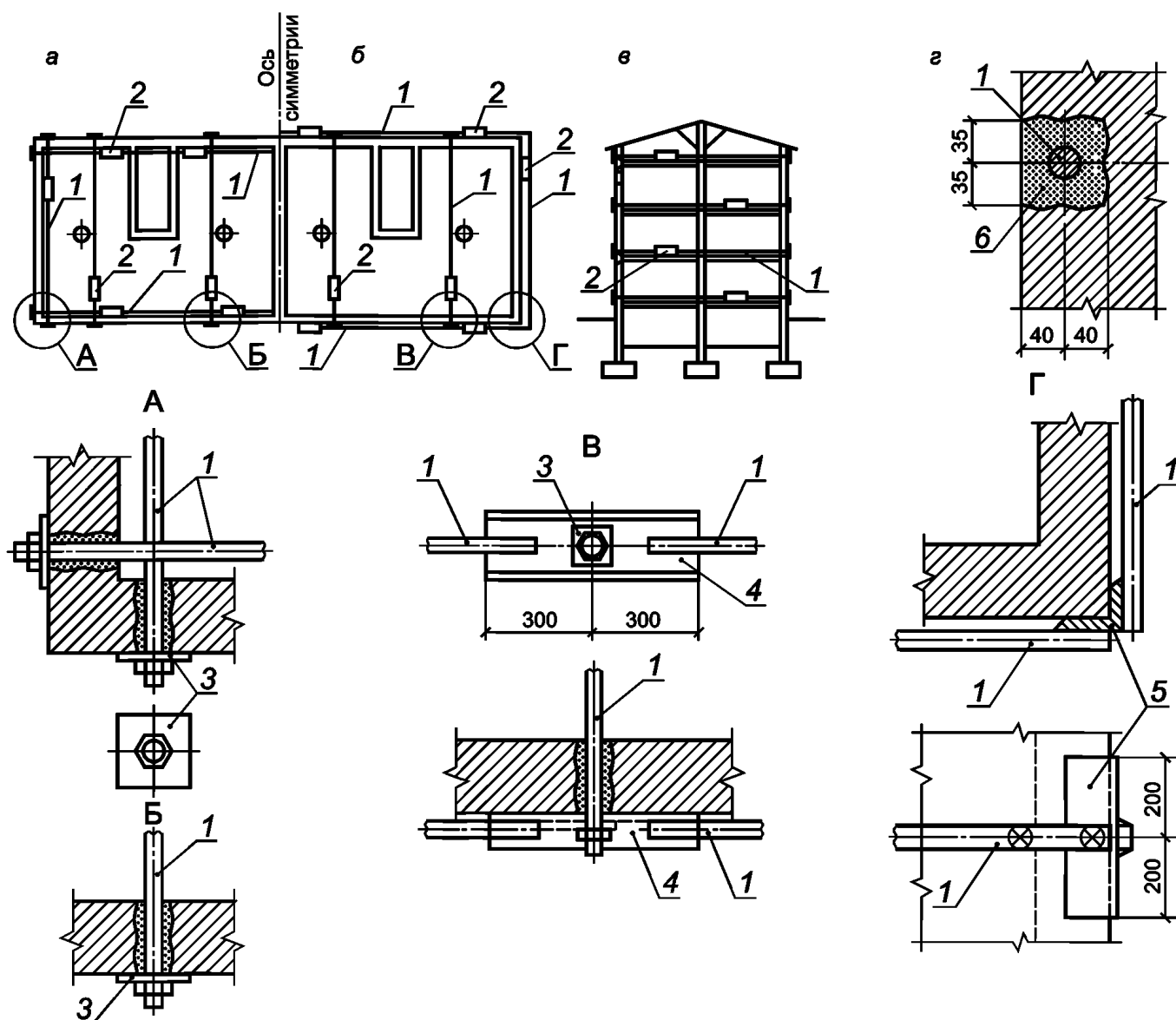
а — внутри здания; б — снаружи здания; в — разрез; г — вариант укладки тяжей в штрабу; 1 — тяж; 2 — муфта натяжения; 3 — металлическая подкладка; 4 — швеллер №16–20; 5 — уголок; 6 — цементный раствор марки М100
