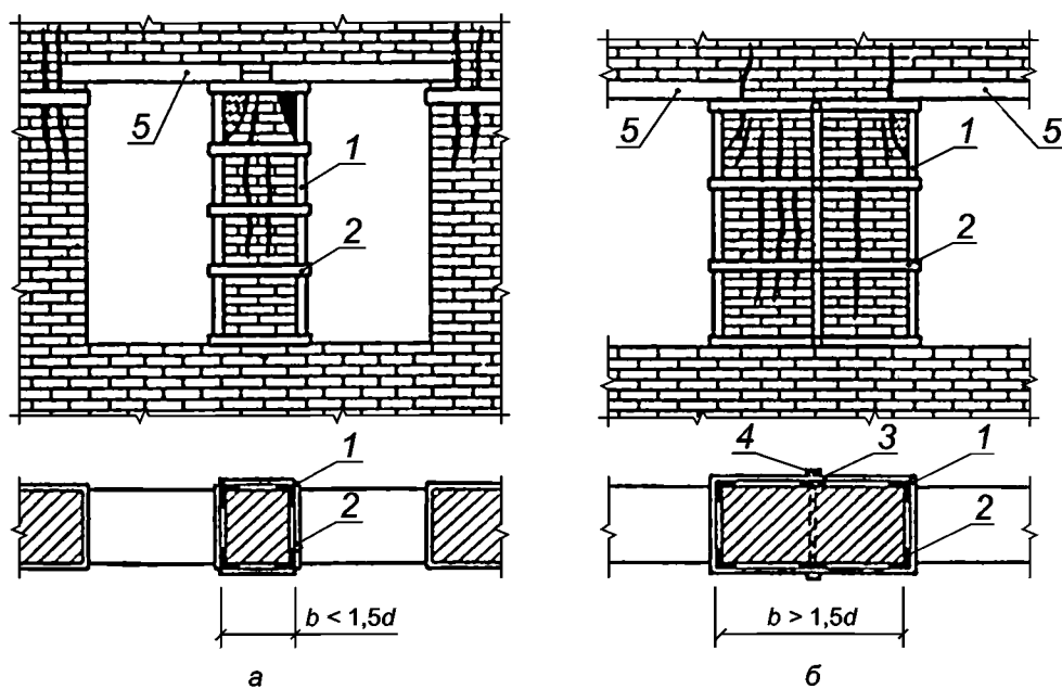
а — при ширине простенков b < 1,5d ; б — то же при b > 1,5d ; 1 — уголок; 2 — планка; 3 — полоса; 4 — болт; 5 — перемычка
