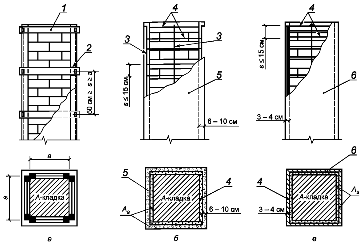
а — металлическая обойма; б — железобетонная; в — армирование штукатуркой; 1 — планка f_1 сечением 35×5 — 60×12 мм; 2 — сварка; 3 — стержни диаметром 5—12 мм; 4 — хомуты диаметром 4—10 мм; 5 — бетон класса В7,5—В25; 6 — штукатурка (раствор марки 50—100)
