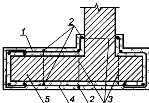
1 — металлическая сетка; 2 — дополнительные стержни, расположенные сверх сетки; 3 — хомуты (связи); 4 — бетон облоймы; 5 — кладка стены
