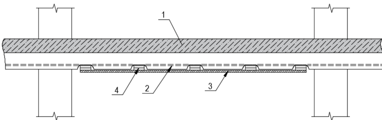
1 – усиливаемая конструкция; 2 – существующая арматура; 3 – дополнительная арматура; 4 – планки или корытчики из арматурной стали
