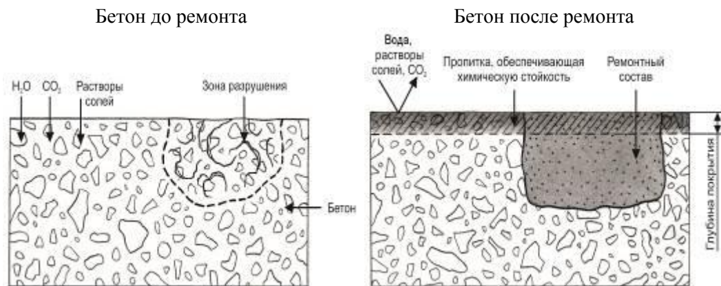
Рисунок Е.2 – Схематическое изображение метода 6.2 до и после применения
