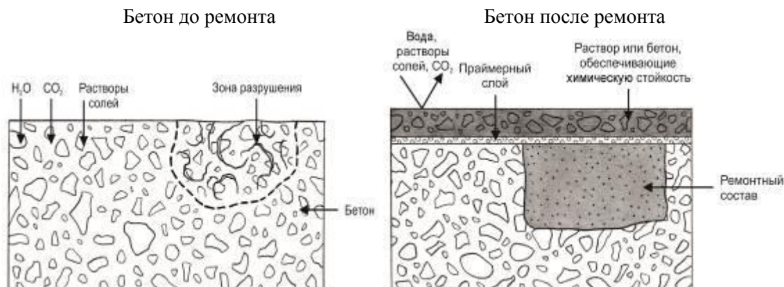
Рисунок Е.3 – Схематическое изображение метода 6.3 до и после применения
