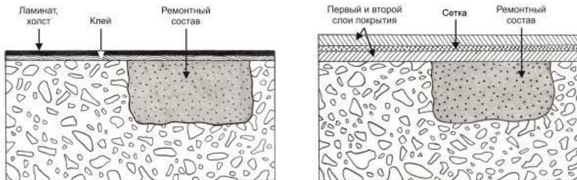
Рисунок Г.6 – Схематическое изображение метода 4.3 до и после применения
