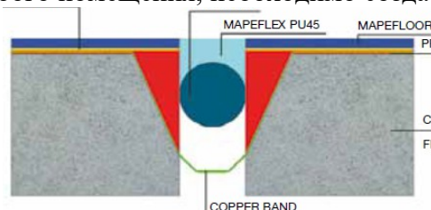
Рис 1. Расположение ленты Copper Band в шве.
